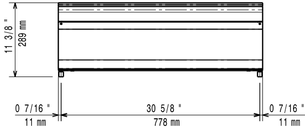
侧视
