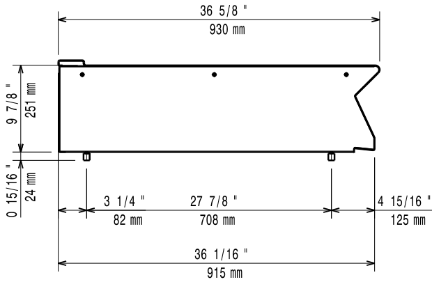
侧视
